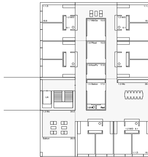
2. Obergeschoss
