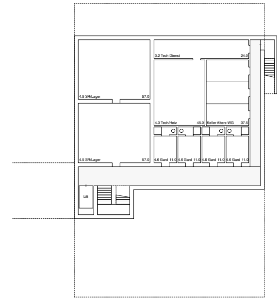
Untergeschoss
