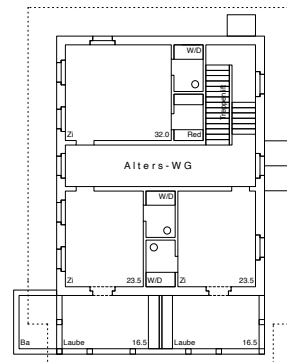
1. Obergeschoss Alters-WG
