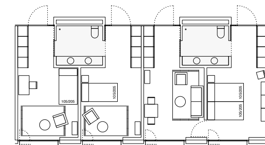
Möblierung Variante Einzelzimmer 1:100 Möblierung Variante Doppelzimmer 1:100
