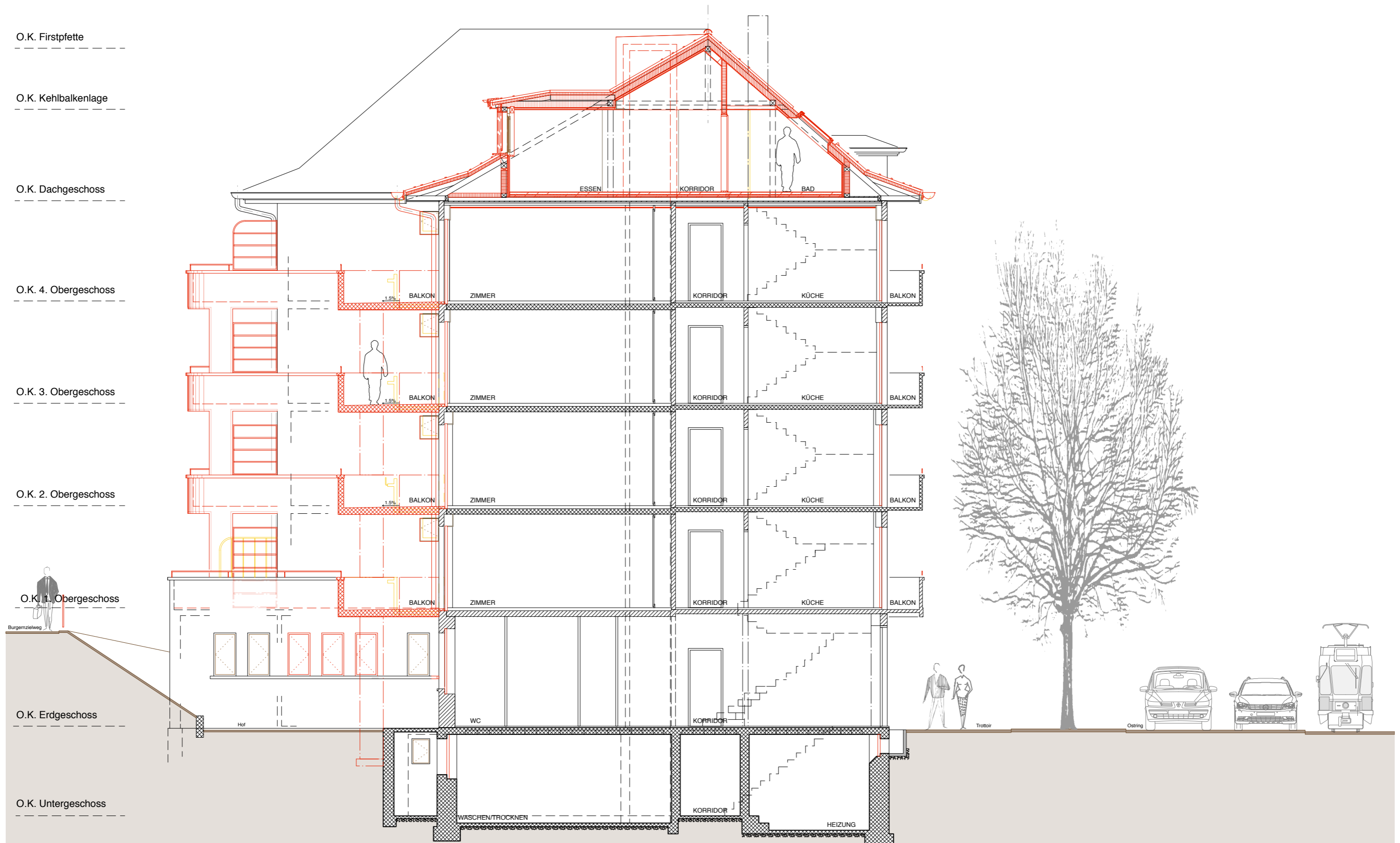
Schnitt A-A
