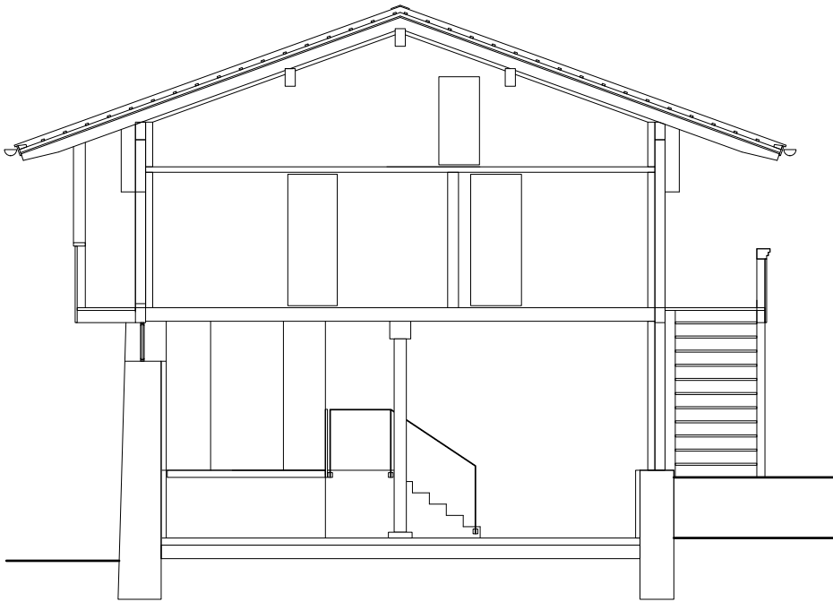
Schnitt A-A
