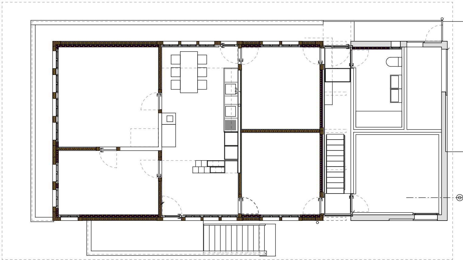
Grundriss Obergeschoss
