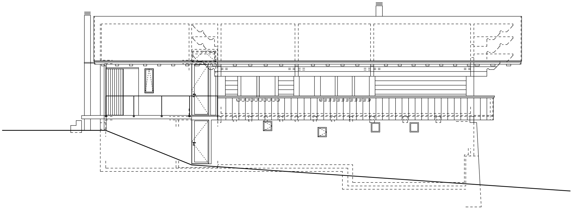
Fassadenansicht West
