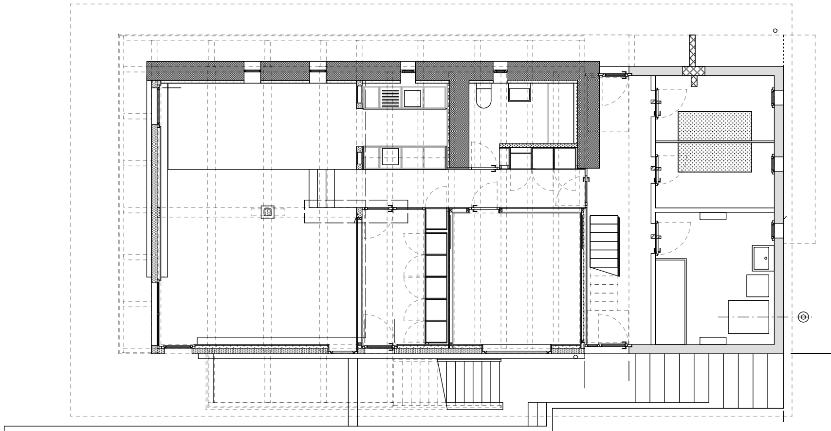
Grundriss Erdgeschoss
