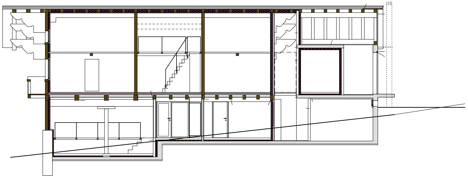
Schnitt E-E
