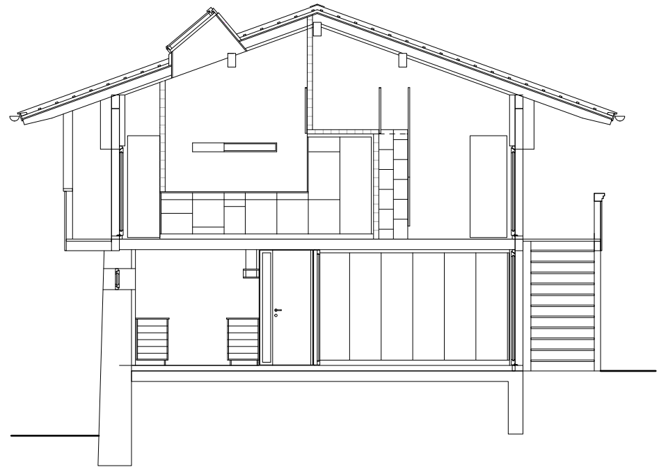
Schnitt B-B
